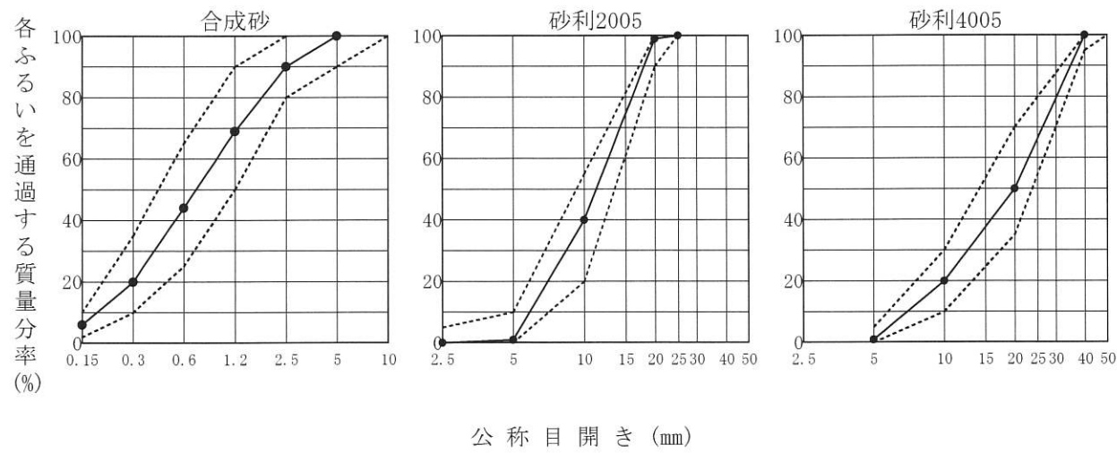
粒度曲線
